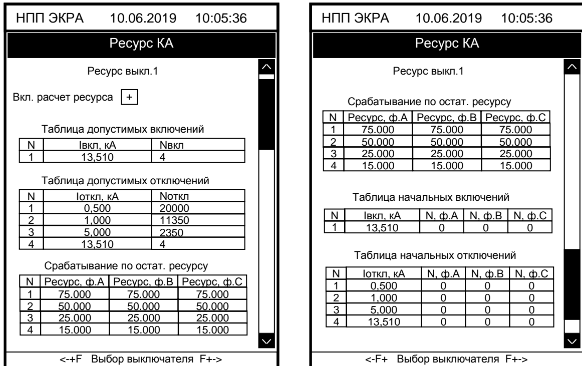
Рисунок 14 – Внешний вид меню Ресурс КА
