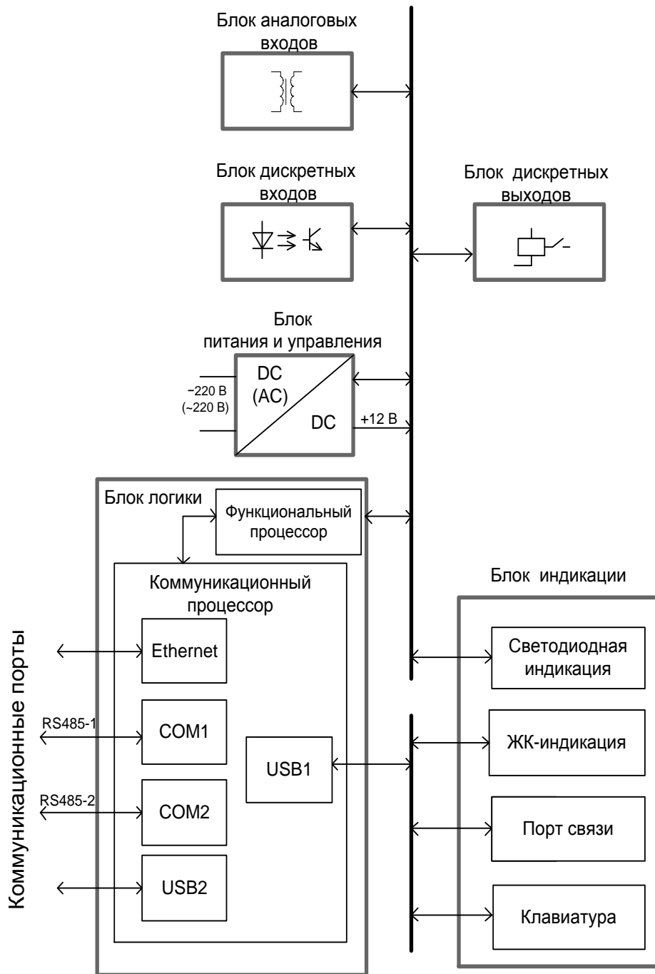
Рисунок 70 – Блок-схема терминалов типов ЭКРА 2Х1(А), ЭКРА 2Х2(А), ЭКРА 2Х3(А), ЭКРА 2Х7(А)
