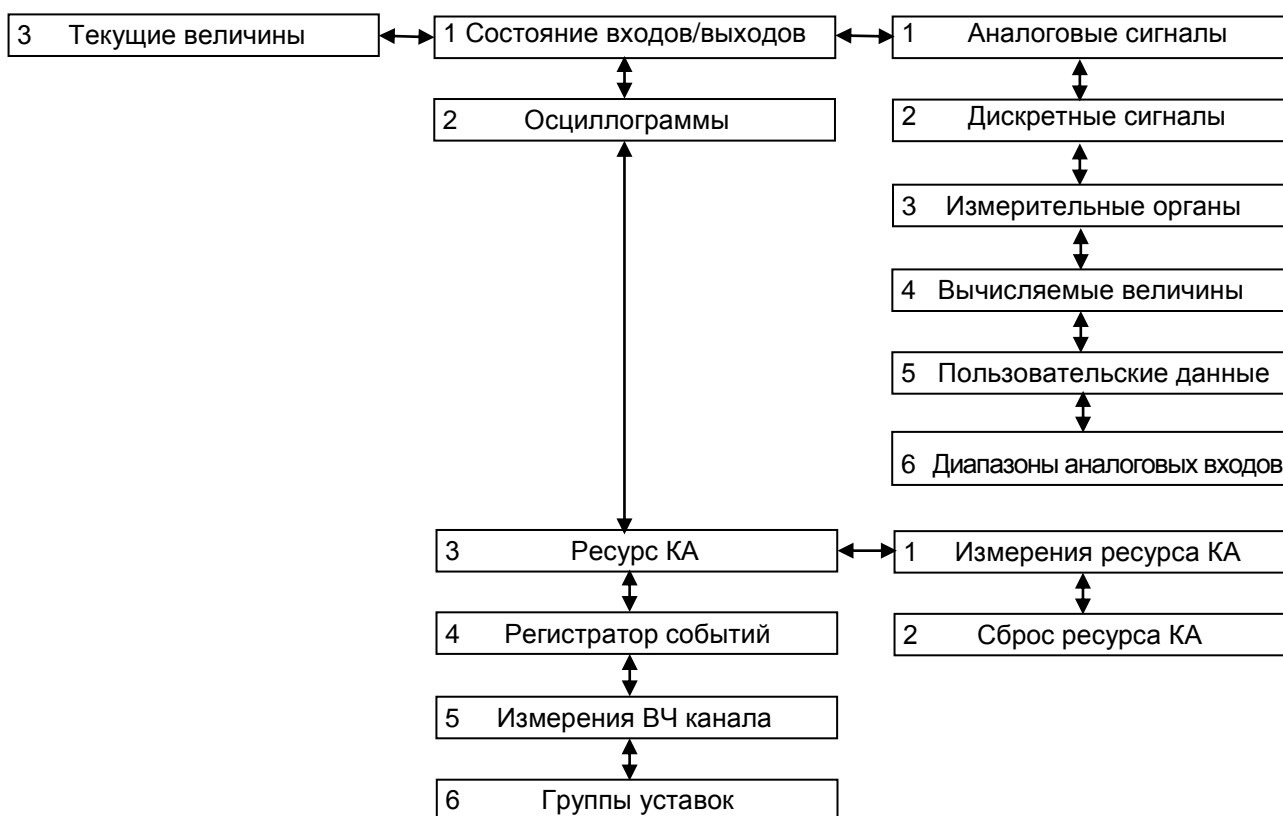
Рисунок 49 – Структура меню Текущие величины
