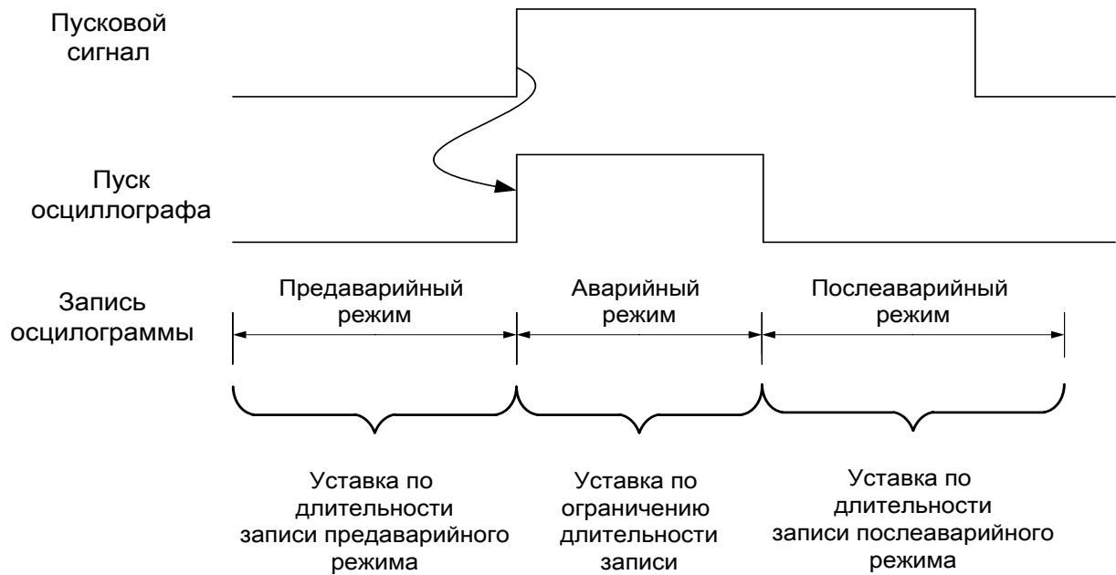
Рисунок 1 – Диаграмма формирования осциллограммы при длительном пусковом сигнале
