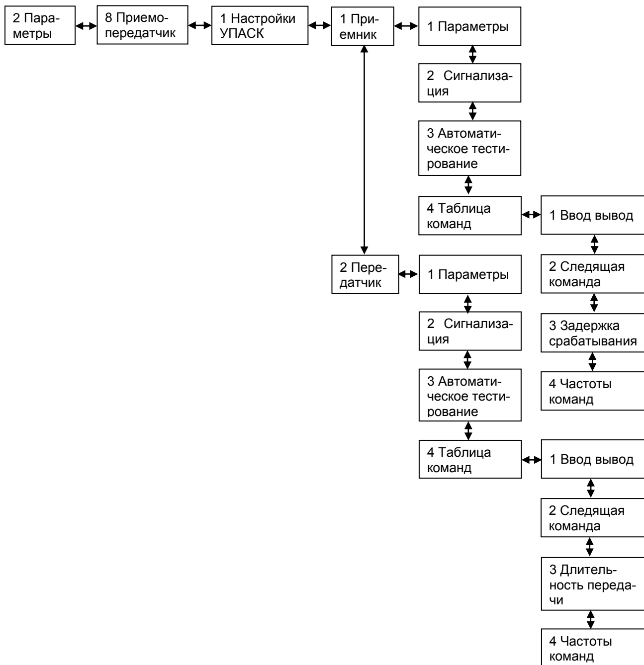
Рисунок 47 – Структура меню Системные параметры
