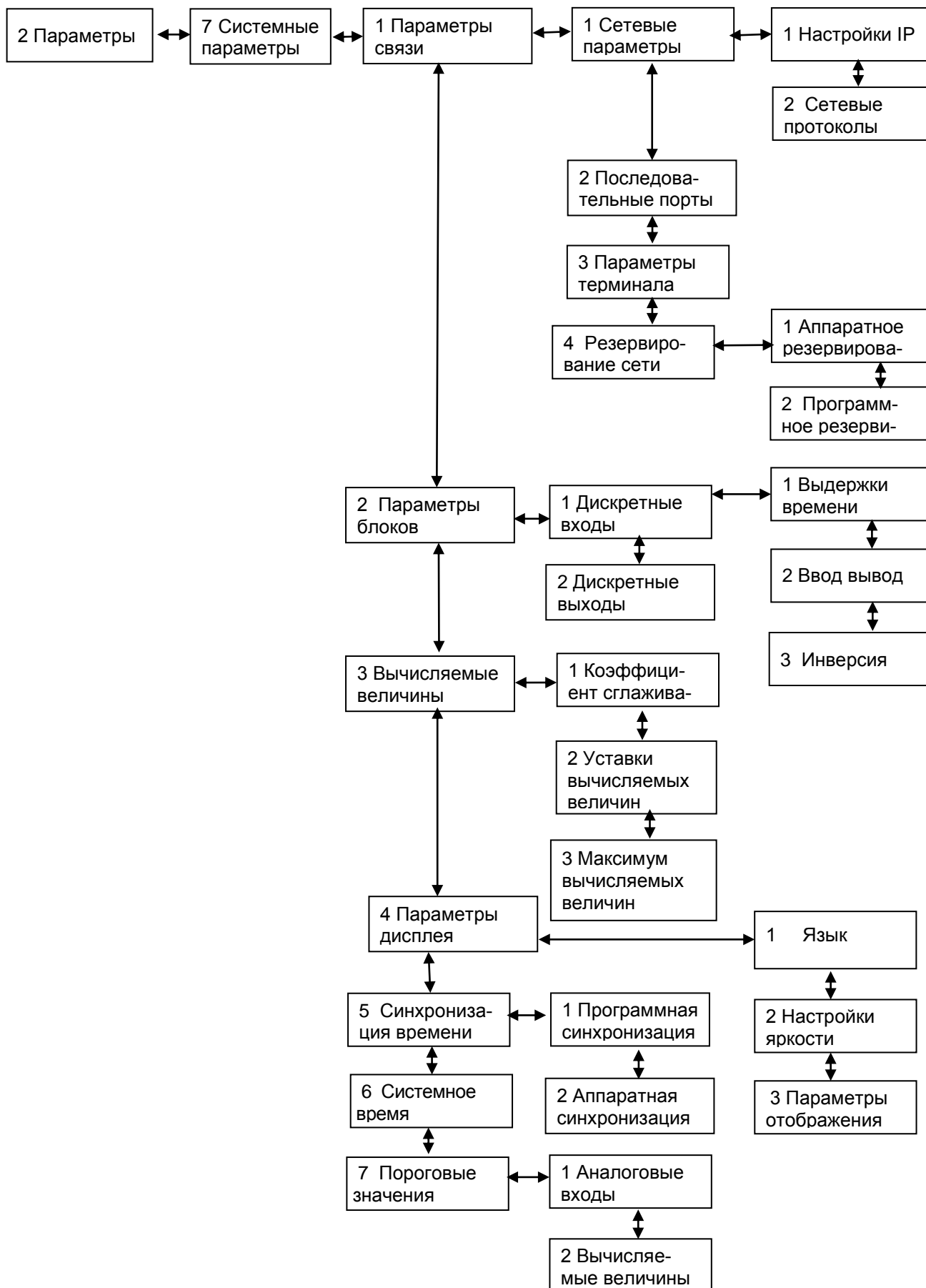
Рисунок 34 – Структура меню Системные параметры
